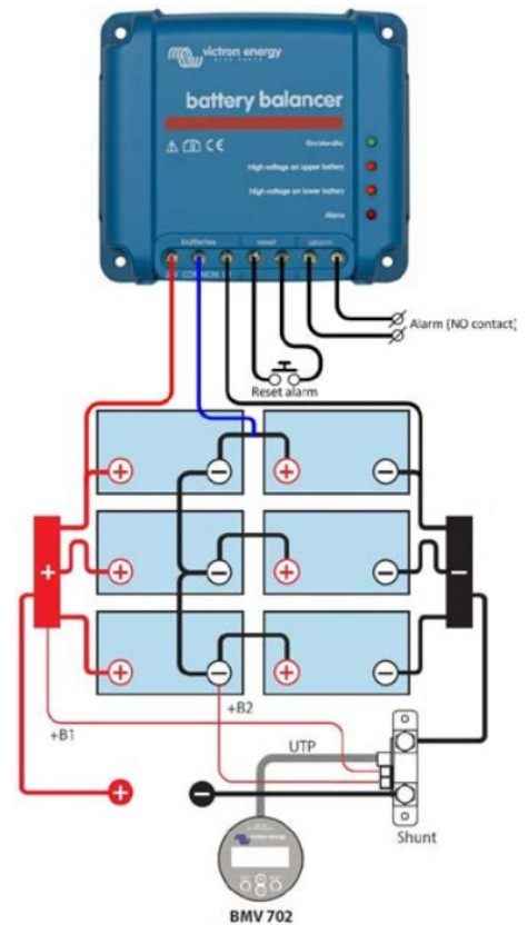
Wyrównywacz akumulatorów podłączony do sześciu akumulatorów 12 V połączonych szeregowo-równolegle (system 24 V)
